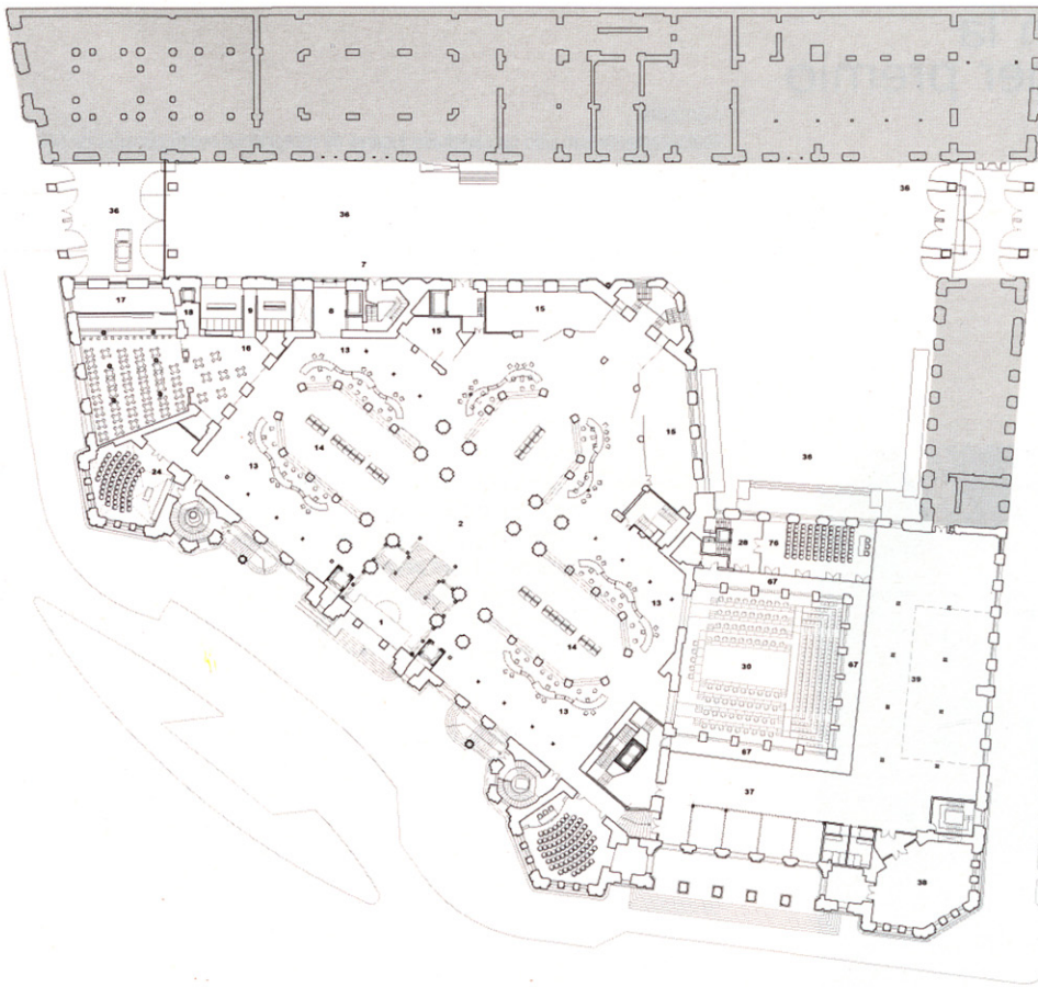
PLANTA SEGUNDA
